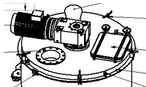
DEMONTAGE RAPIDE DU COUVERCLE
