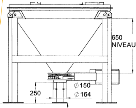
VANNE ELECTROPNEUMATIQUE * DN150
